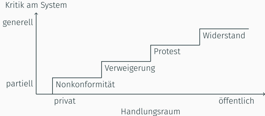
Abbildung 6: Stufenmodell des abweichenden Verhaltens nach Detlev Peukert
